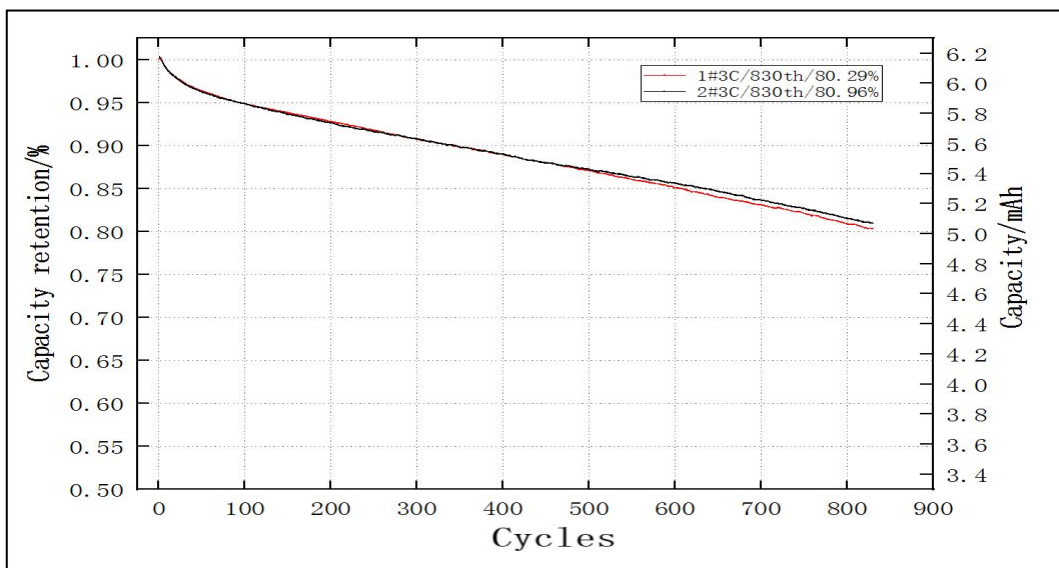
6.0 Ah 磷酸铁锂电池 30±2℃ 3C 循环曲线图 30±2℃ 3C cycle curve of 6.0 Ah LiFePO 4 cell
