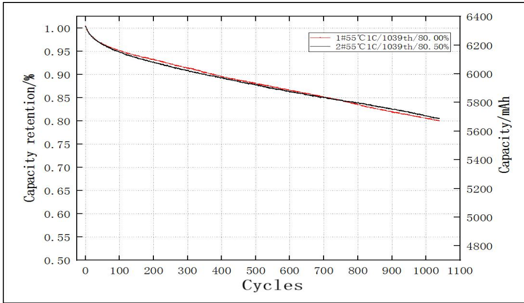
6.0 Ah 磷酸铁锂电池 55±2℃ 1C 循环曲线图 55±2℃ 1C cycle curve of 6.0 Ah LiFePO 4 cell
