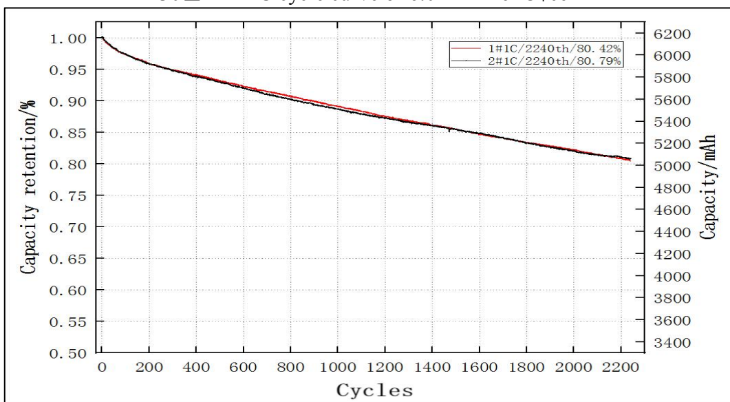
6.0 Ah 磷酸铁锂电池 30±2°C 1C 循环曲线图 30±2°C 1C cycle curve of 6.0Ah LiFePO 4 cell
