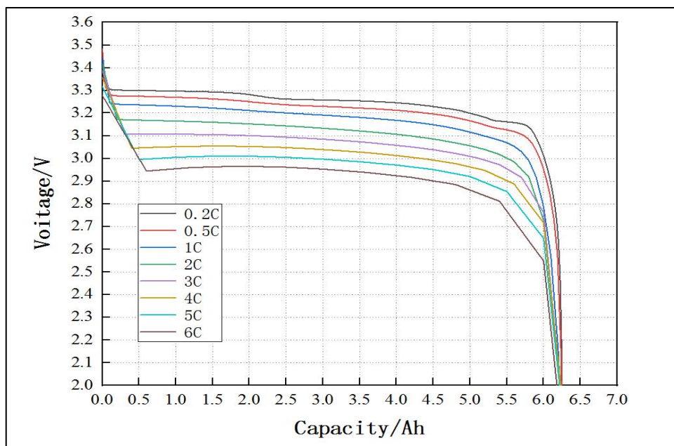
6.0Ah 磷酸铁锂系电池不同倍率放电曲线 Different rate discharge curve of 6.0Ah LiFePO 4 cell
