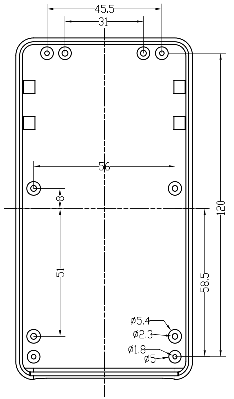
上盖底视图
